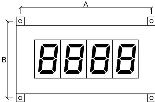
(Standard Type) 256(W) X 126(H) X 65(D) mm Hole Size : ( A:231(281) B:151(101) mm )
