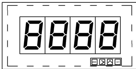
(Panel Type) 260(W) X 140(H) X 65(D) mm
