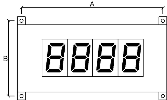
(Local Type) 300(W) X 170(H) X 80(D) mm Hole Size : ( A : 270(330) B : 200(140) (mm) )
